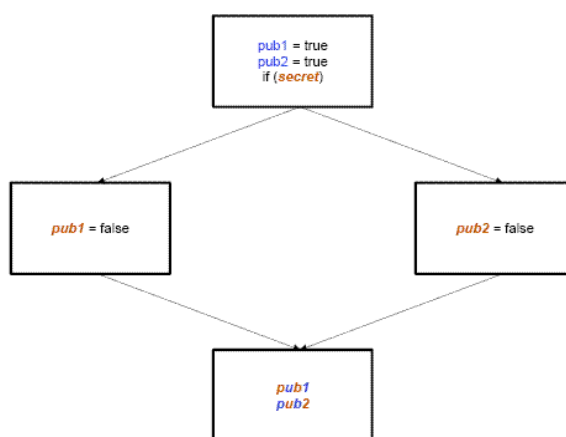
Fig. 1. Flujo de información implícito de secret a pub1 y pub2
