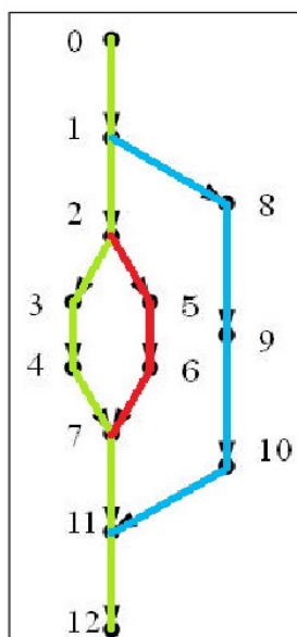
Fig.3. Ejemplo de CFG
