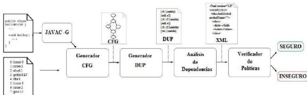
Fig. 2. Secuencias de acciones de la herramienta.
