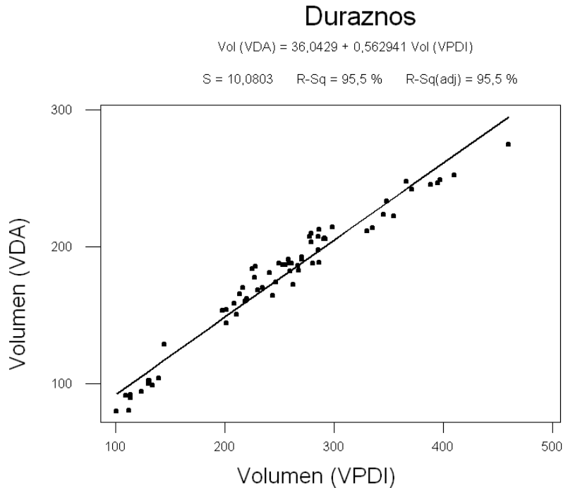
Fig. 8 – Modelo de Regresión simple para la estimación de volumen de Duraznos
