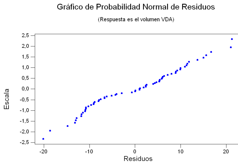
Fig. 9 – Gráfico de Probabilidad Normal para Residuos de la muestra de Duraznos
